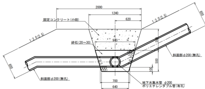
地下水集水管 \phi 200
