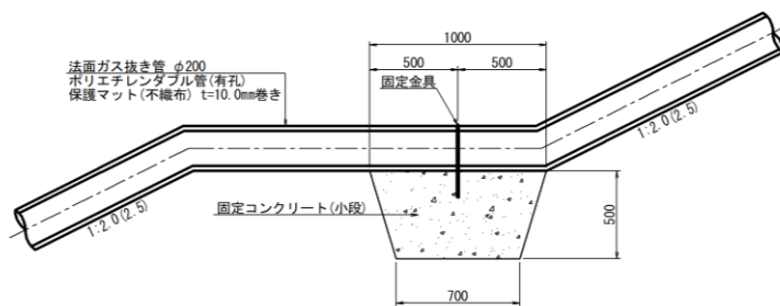
法面ガス抜き管 \phi 200
