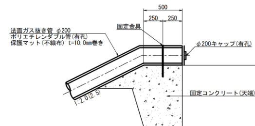
法面ガス抜き管 \phi 200
