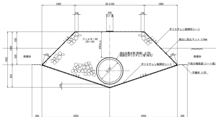
浸出水集水管 (幹線) \phi 700
