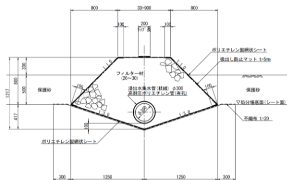
浸出水集水管 (枝線) \phi 300
