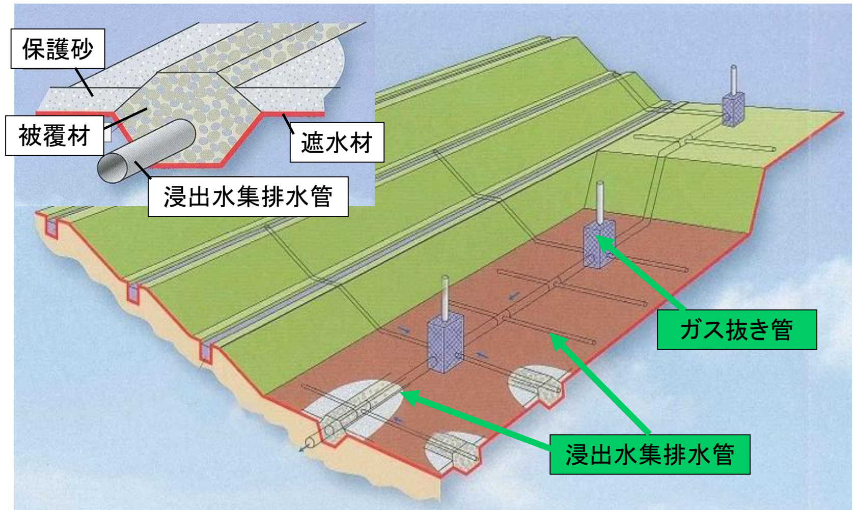
浸出水集水設備の構造
