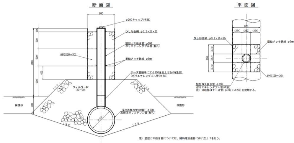
縦型ガス抜き管 \phi 200
